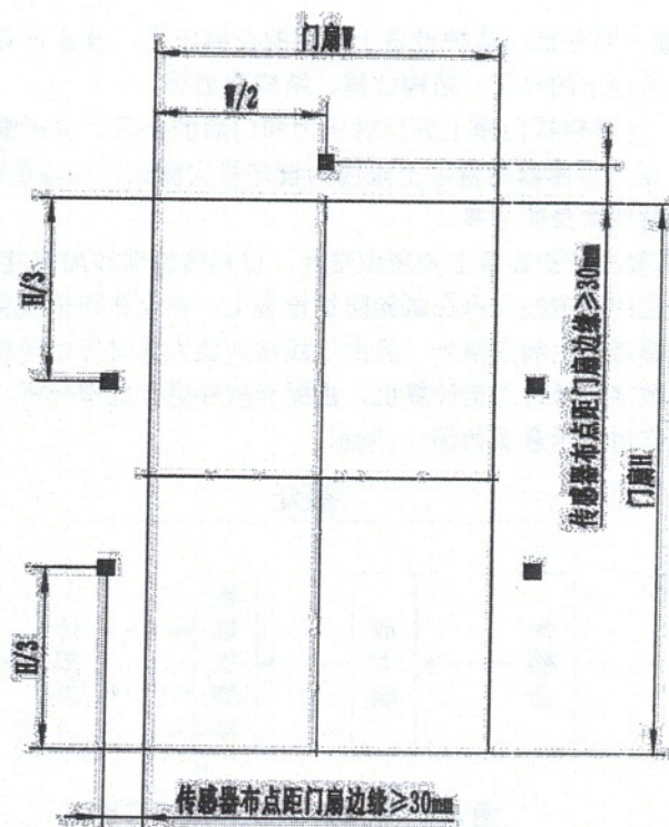
图A.4 传感器布点示意图
