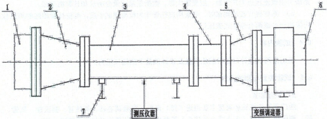
图 G.1 通风性能试验装置示意图
