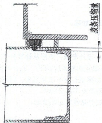
图1 挤压式
