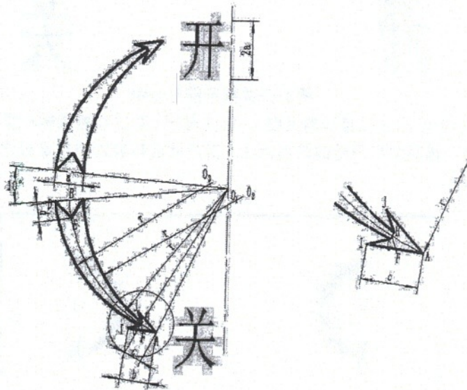
图5 开关指示箭形标志尺寸示例
