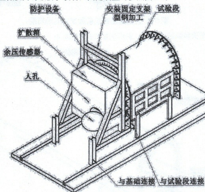
图B.1 小型防护设备固定方式示意图
