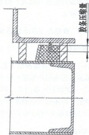
图2 嵌压式
