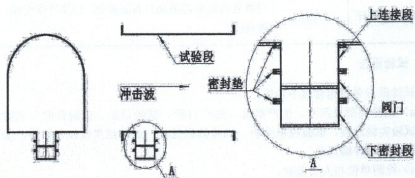
图 B. 4 阀门固定方式示意图
