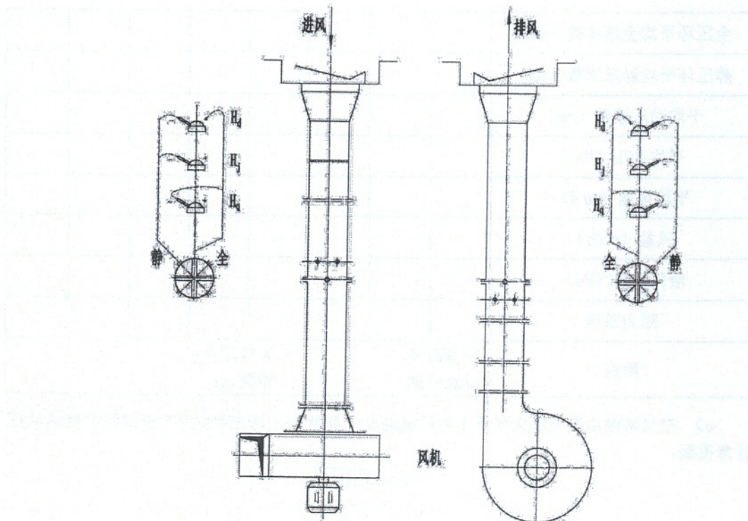
图 G.2 通风性能试验测试系统连接图
